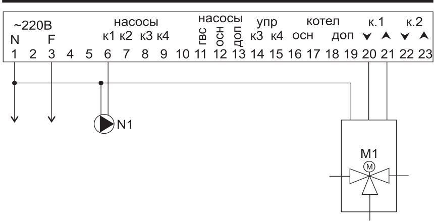
Рис.2.10. Электрическая схема подключения элементов контура.
