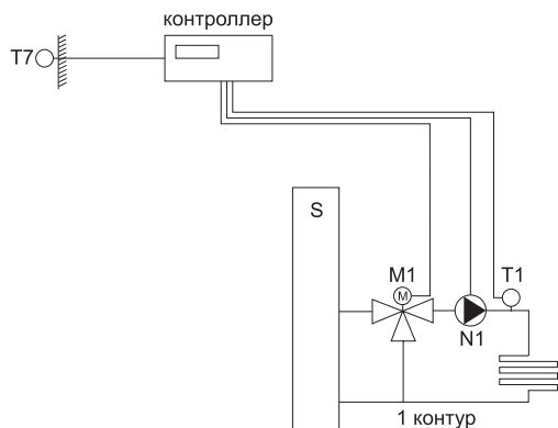
Рис. 2.9. Схема управления контуром
