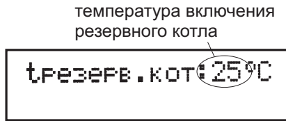
Рис.4.5. Экран настройки температуры включения «резервного» котла
